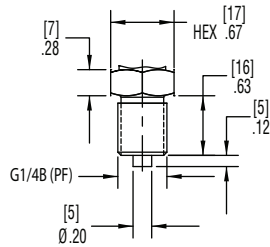
G1/4B (PF) Optional
