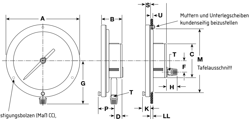
8 1/2" Anschlusslage unten
